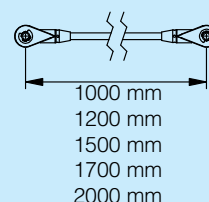
Tension rod
